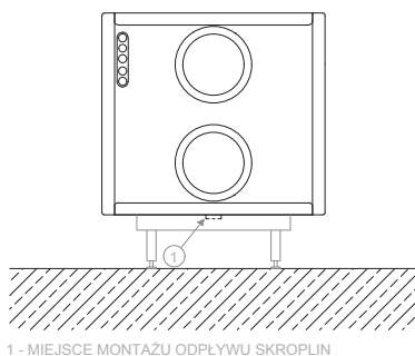
Konsola do montażu urządzenia na podłodze
