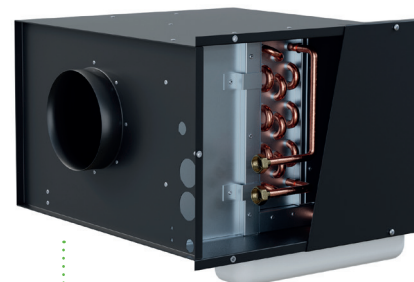
Kanałowa chłodnica wodna
