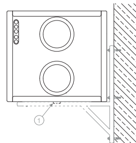
Zestaw wsporników do montażu urządzenia na ścianie
